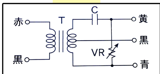
【側面回路図】
